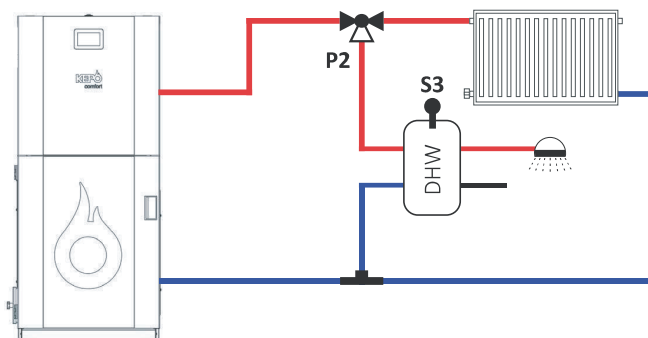
Šema 2 (P26=2)
