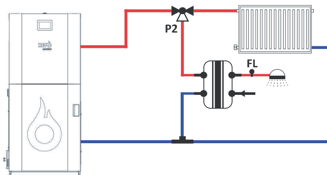
Šema 0 (P26=0)
