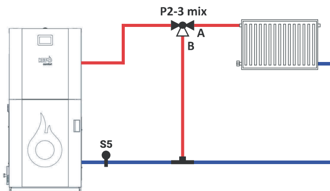
Šema 7 (P26=7)
