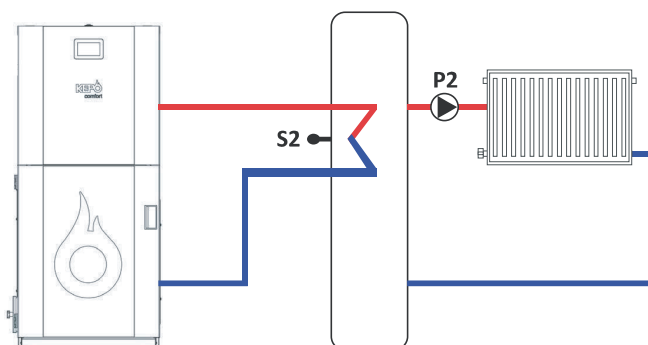
Šema 4 (P26=4)
